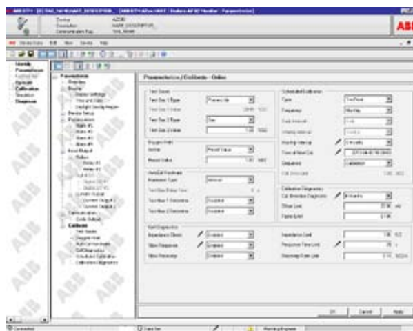
Графический интерфейс
